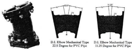
D. I. Elbow MJ/MJ 22.5 degree
