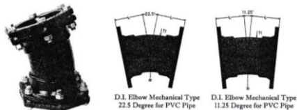
D. I. Elbow MJ/MJ 22.5 degree
